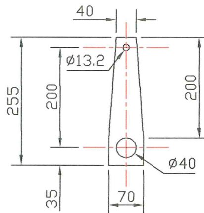
DETAIL PALONNIER PILOTE
