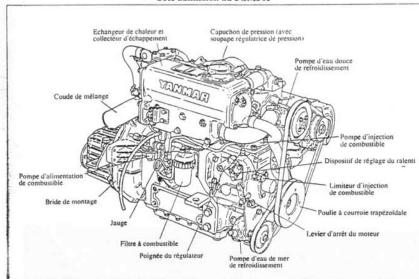
Côté échappement du 3GM30F
