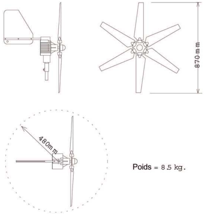
Plan dimensionnel
